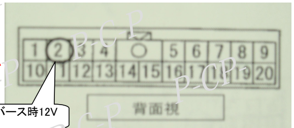
コネクタ①形状・配線
