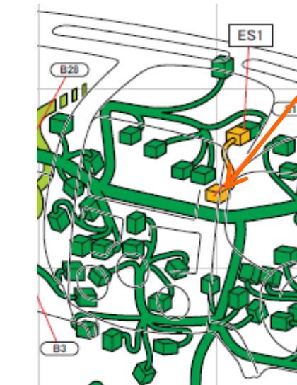
S1 乳白色コネクタ(ナビ、オーディオ部コネクタ)
