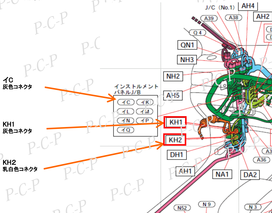
KH2コネクタ
