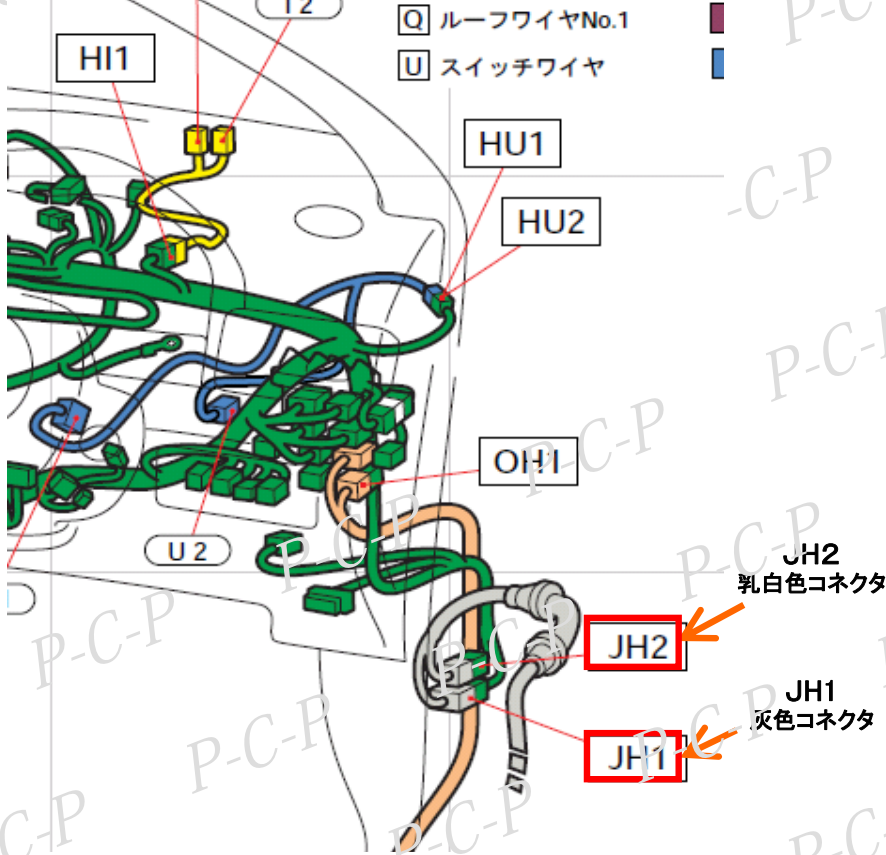
JH2コネクタ
