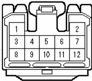
JH1コネクタ
