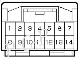
JH2コネクタ
