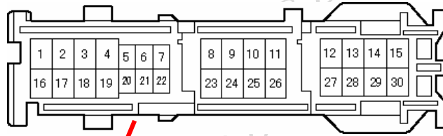
IAコネクタ
