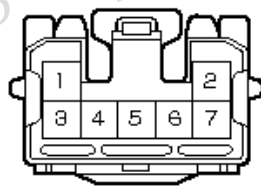
JH1コネクタ
