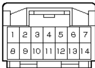
KH2コネクタ
