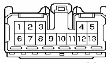
BG1コネクタ
