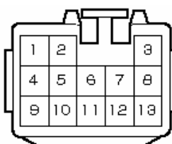
KG2コネクタ
