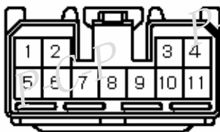
JG2コネクタ
