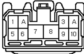
ICコネクタ
