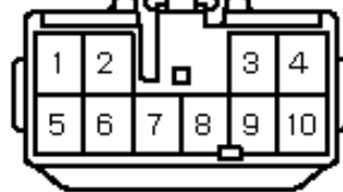
G26コネクタ
