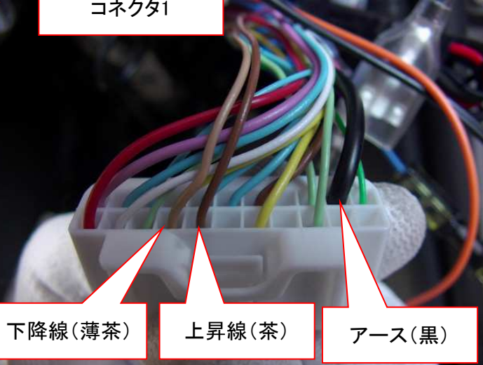
コネクタ1
