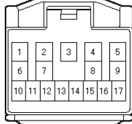
J/B内 イムコネクタ
