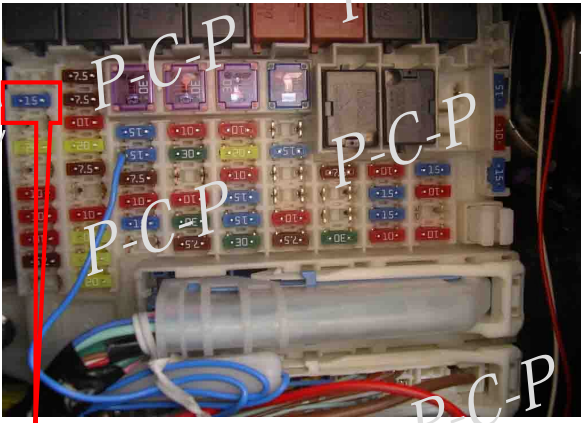
ヒューズボックス内、15A“バックアップ”より電源取出ヒューズにて接続。
