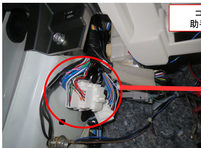
リバース時+12V (ピンク)
