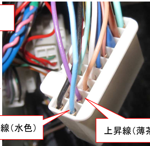
コネクタ3 ナビ裏20ピンコネクタ
