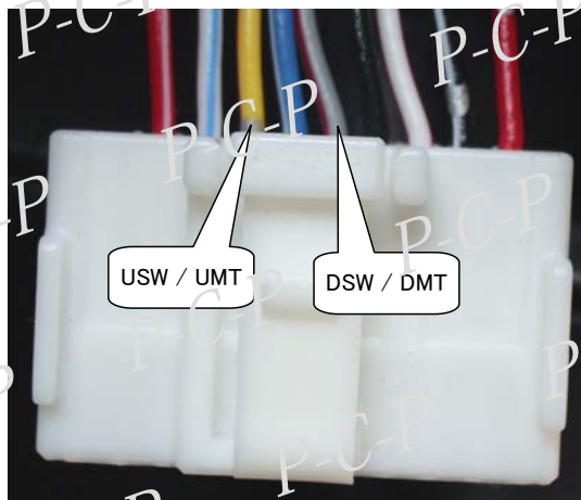
ドアミラースイッチコネクタ
