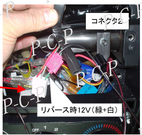
結線しやすいようオーディオ側からコネクタの配線留めを外す 写真手前側配線留め (コネクタ2, 3用参考写真)
