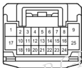
IE2コネクタ
