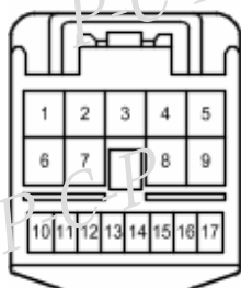
IE1コネクタ
