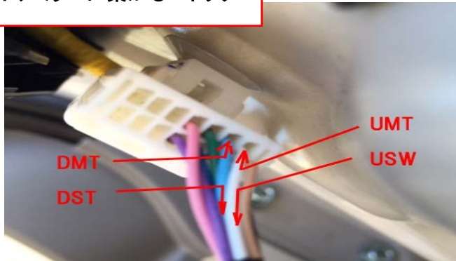
コネクタ1 運転席ドアパネル内ドアミラーに繋がるコネクタ
