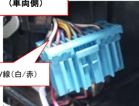
オーディオコネクタ (車両側)
