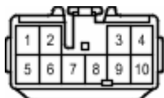
E32(ナビ裏コネクタ)
