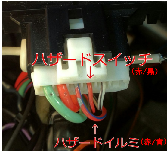
コネクタ 2
