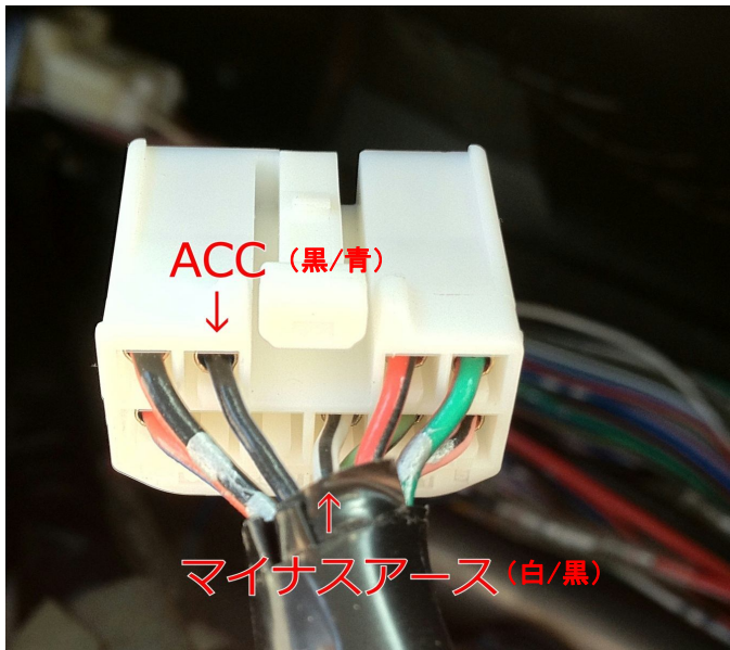
コネクタ 1
