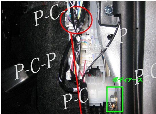
運転席足元
