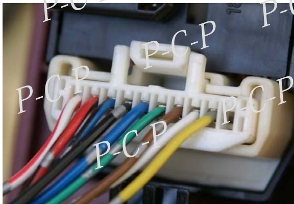
コネクタ1拡大
