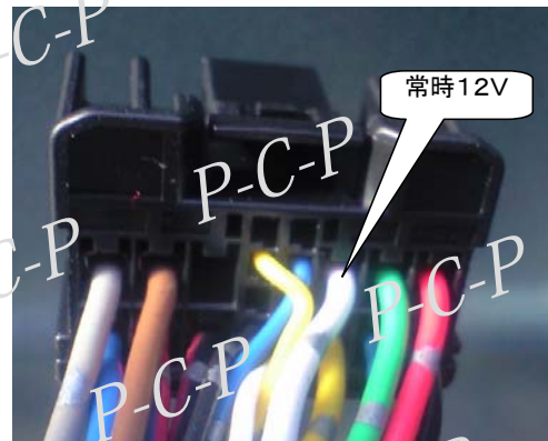
コネクタ2 パワーウインドー接続コネクタ
