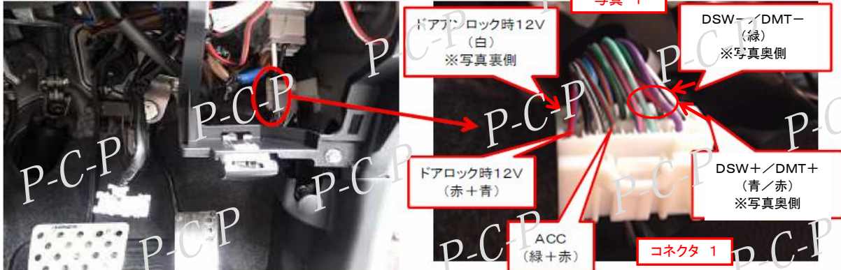
■コネクタ1(運転席キックボード内、灰色コネクタ裏)
