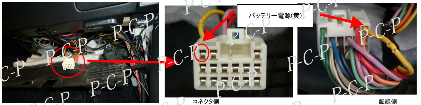
コネクタ3 運転席側ヒューズ裏のサービスコネクタ
