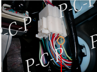
ドアロック時一瞬+12V (No17)
