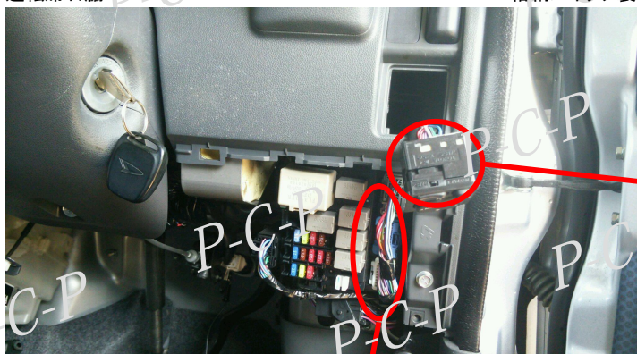
格納スイッチ裏
