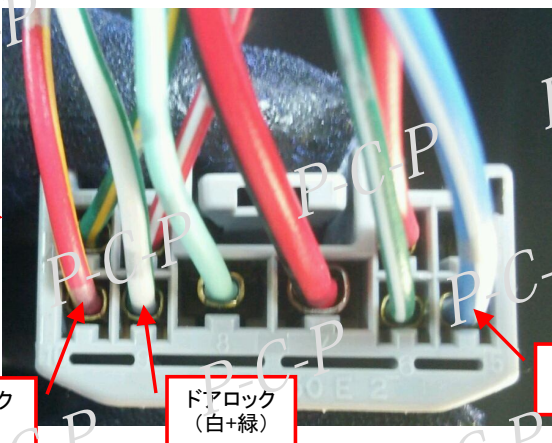
コネクタを外してツメを上にした状態
