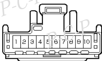
D52コネクタ
