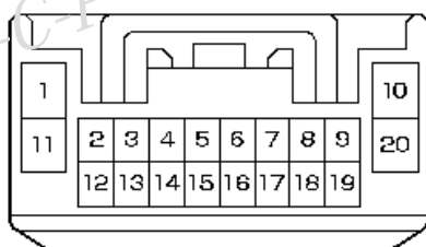
FD1コネクタ
