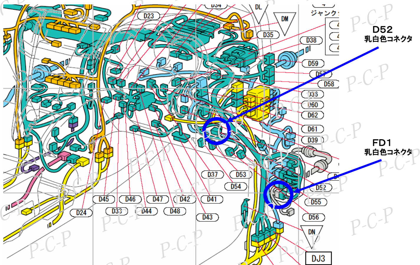
D52コネクタ
