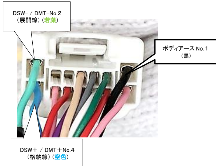
コネクタ 1 運転席ドア内部 (ミラースイッチ裏コネクタ)
