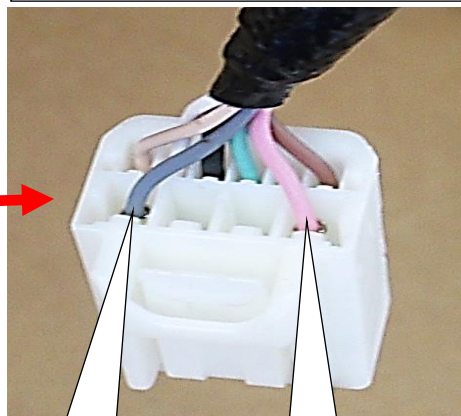
ドアアンロック時 一瞬+12V (灰)
