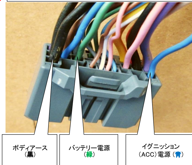
コネクタ 3 運転席ドア内部 (パワーウィンドースwitch裏コネクタ)
