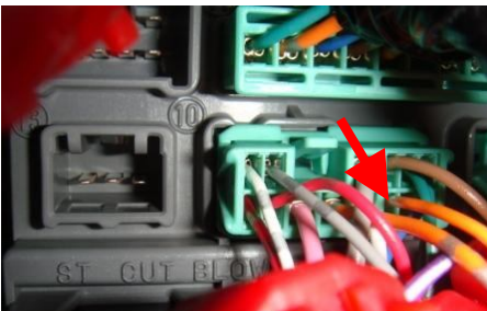
コネクタ5 ヒューズボックス最下段左端付近
