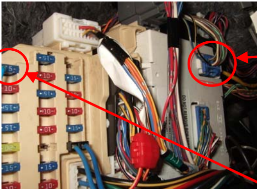
コネクタ1 ヒューズBOX部
