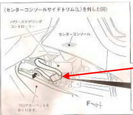
コネクタ4 センターコンソールトリム内
