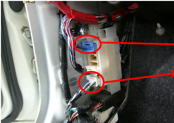
助手席足元
