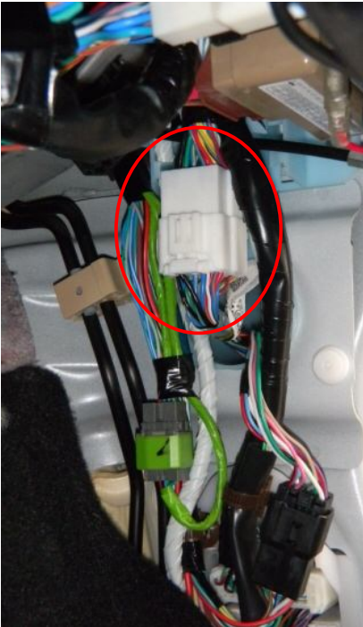
コネクタ2の情報(運転席足元右)
