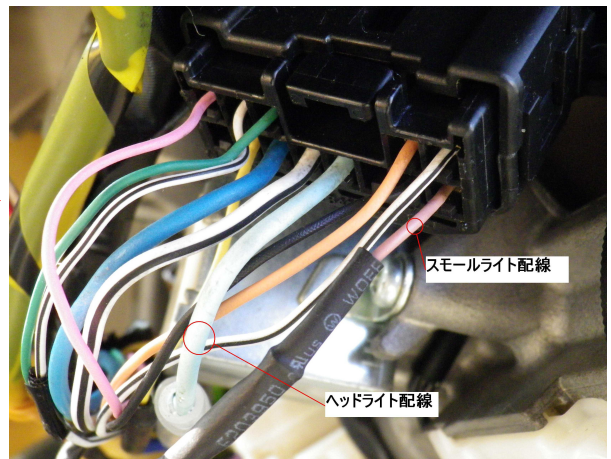
コネクタ1
