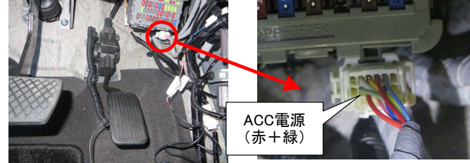
コネクタ2 運転席足元右側、ヒューズボックス下部
