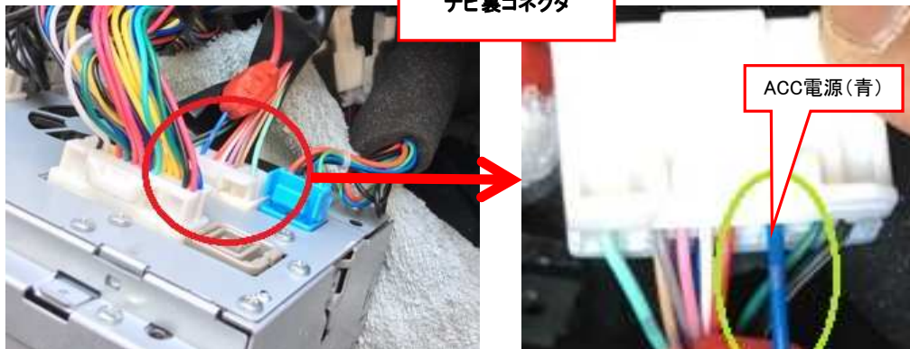
コネクタ1 ナビ裏コネクタ
