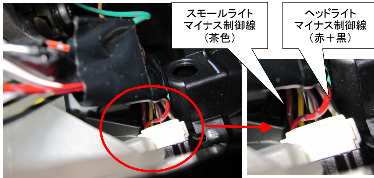
コネクタ2 ライト信号コネクタ
