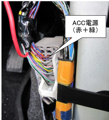
コネクタ1 運転席足元脇
