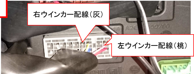
コネクタ3 グローBOX裏
