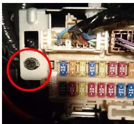
ボディーアースヒューズBOX横ボルト
