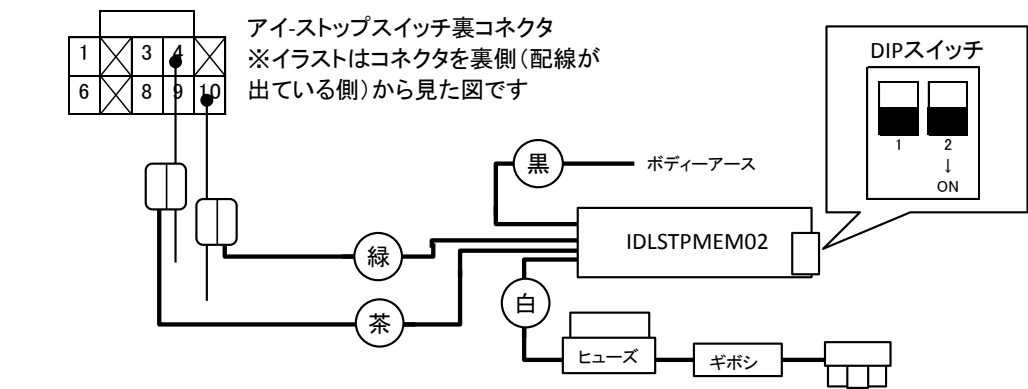
アイストップスイッチコネクタ結線先配線色表
